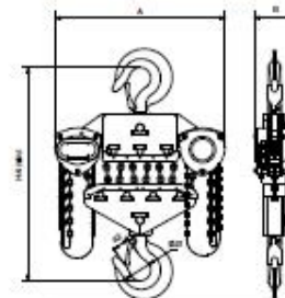
VHR 5, 6 et 8 brins
